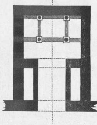
FIG. 5.—Planta de los muros interiores del mausoleo (hoy cripta) de Santiago. Lo marcado con líneas diagonales indica la obra nueva.
