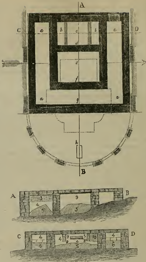
EL SEPULCRO DE SANTIAGO. — PLANTA.— a . Andito, ó galería subterránea.— b . Sepulcros de los discípulos Teodoro y Atanasio, abiertos en el suelo.— c . Lugar sobre que descansaba el sarcófago del Apóstol.— d . Sitio de donde arrancaba el arco de entrada á la cámara sepulcral.— e . Antecámara ó iglesia subterránea.— f . Sitio de donde arrancaba el arco de entrada á esta iglesia por el andito ó galería exterior.— g . Lugar correspondiente al del piso principal, en que aparecía la puerta de entrada al edificio, la cual miraba hacia el Oriente.— h . Local ó repositorio donde se han hallado las reliquias, hacia el extremo oriental del ábside. Las líneas de punto s , que se acerca á las letras a , a , h , corresponden á la planta del altar mayor, labrado entre los años 1650 y 1659.
