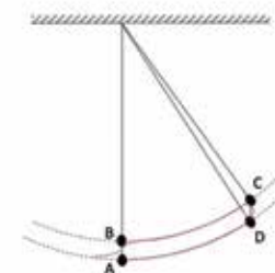
Fig 1 : Mise en mouvement du Botafumeiro : au point A, la corde est retenue de près, ainsi le caisson se déplace de B en C suivant une course avec une longueur de corde réduite. Au point de conversion C, le caisson tombe au point D, le mouvement se prolonge dans une course déterminée par la longueur de corde initiale. En décalage avec la ligne idéale, le mouvement qu'on peut observer en réalité est représenté par la ligne rouge.
