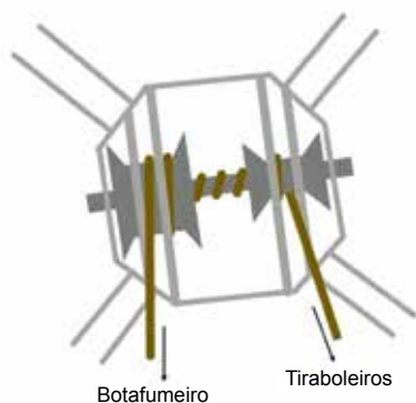
Fig. 2: Schema der Aufhängevorrichtung, Rollen mit Achse fest verbunden, auf Traggestell aufliegend, verankert in Säulen der Kuppel, Seil um Rollen und Achse gewickelt, durch Schienen seitlich gehalten
